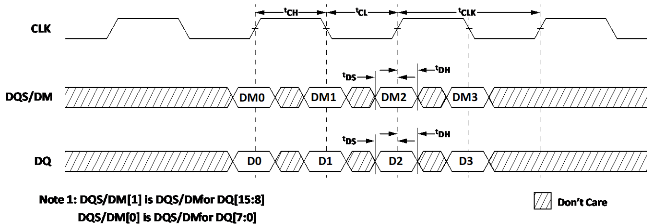
Figure 12: Write DQS/DM & DQ Timing
